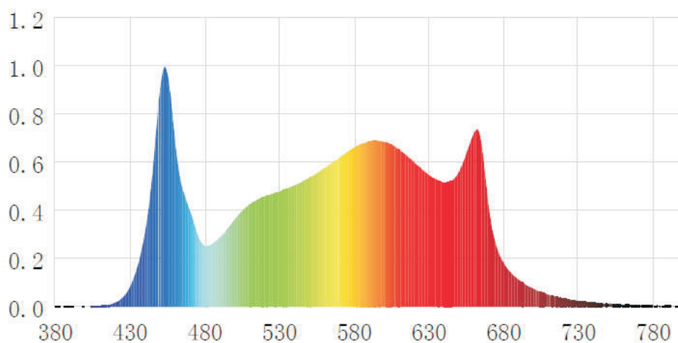
MAXIMUS-2FT 4000K+660nm
