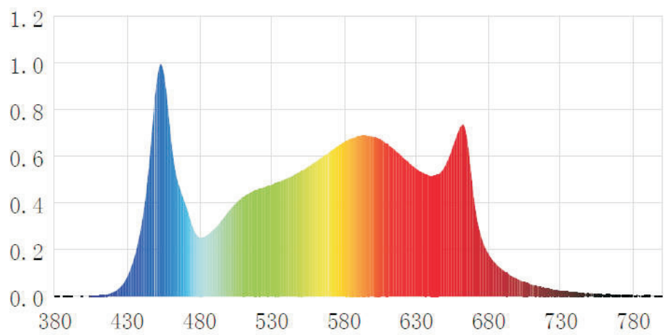
MAXIMUS-4FT 4000K+660nm
